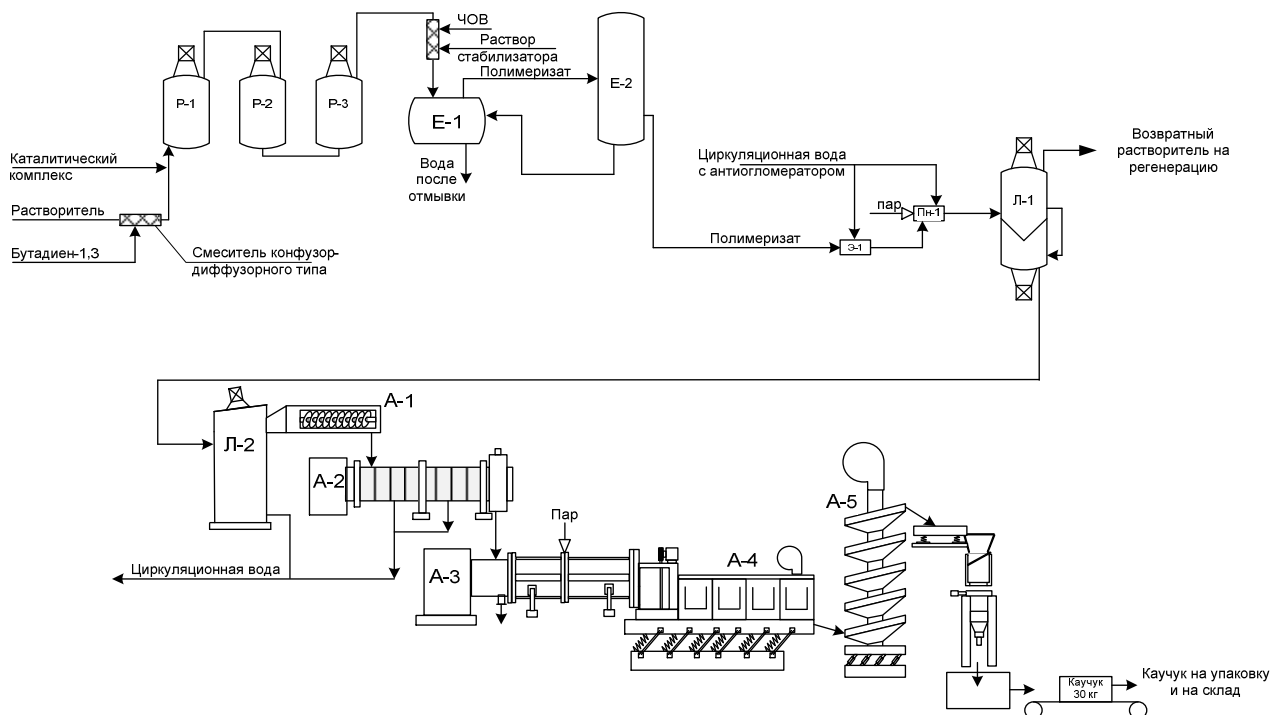
Рисунок 2.1.4 — Схема получения каучука СКДН
