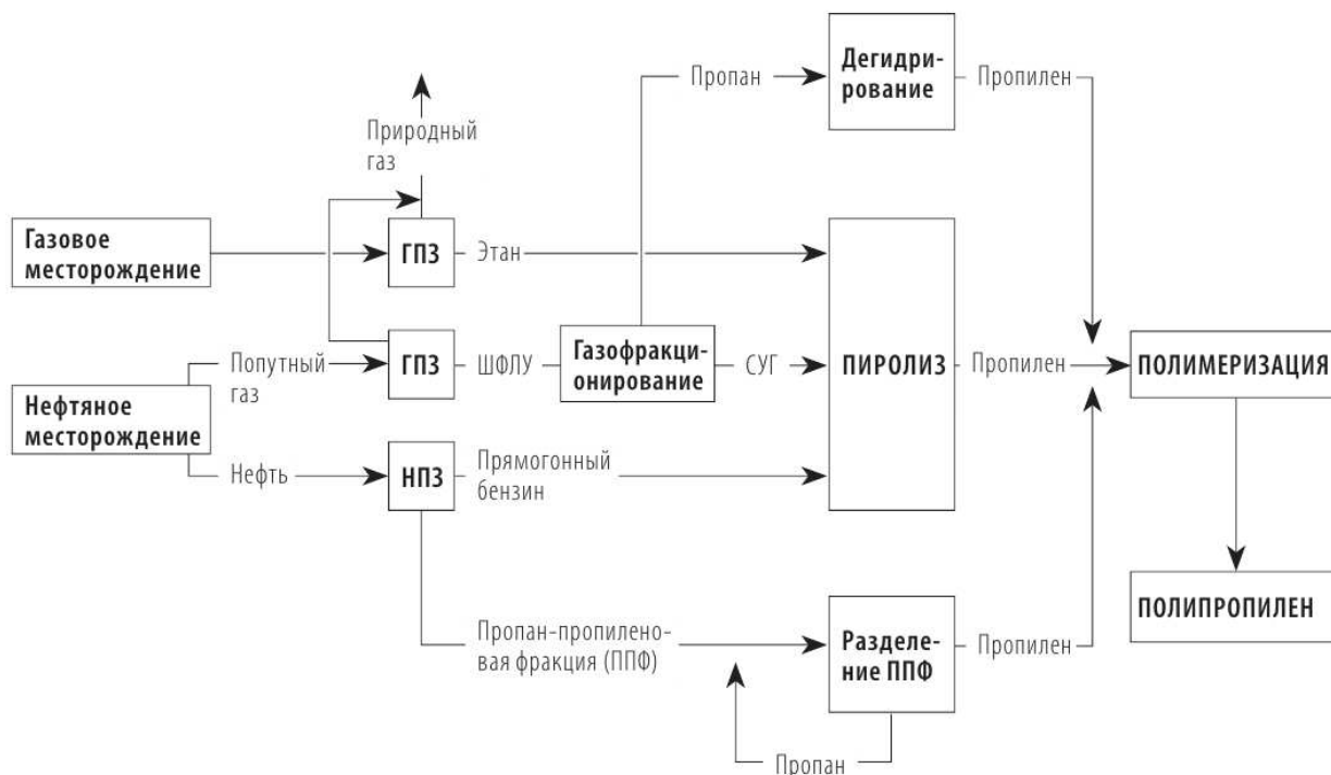
Рисунок 5.3 — Принципиальная схема получения ПП
