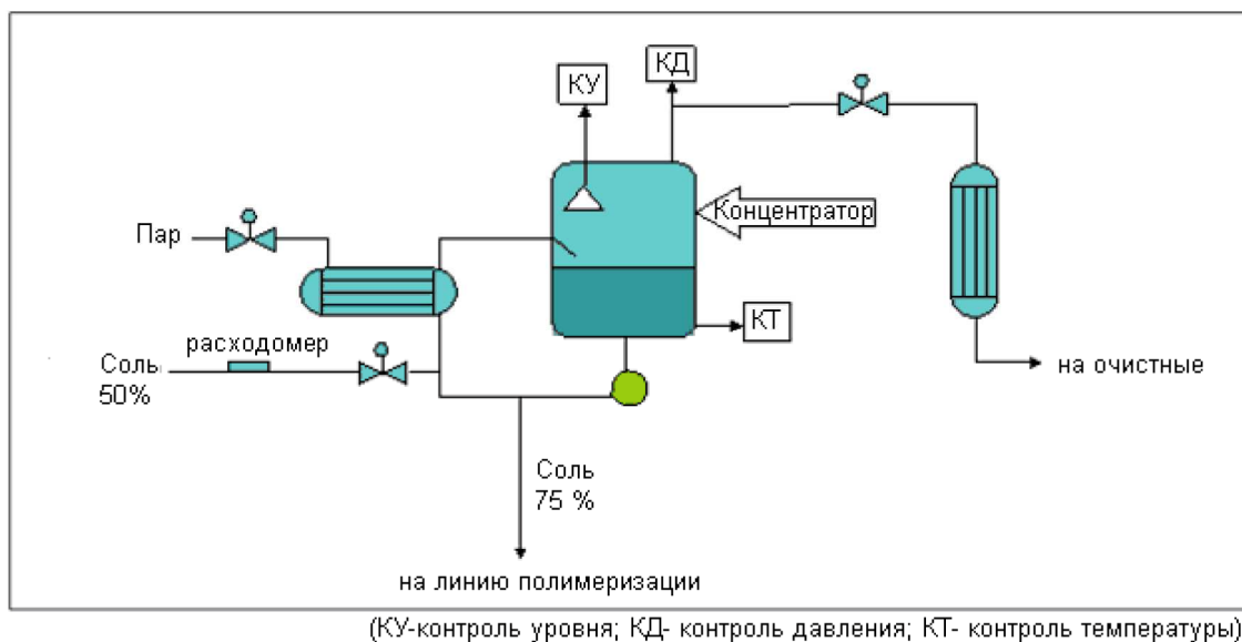
Рисунок 10.2.4 — Блок-схема процесса концентрации соли для производства ПА 66
