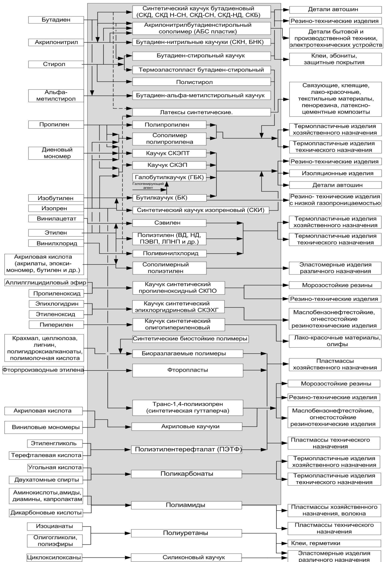
Рисунок 1 — Сфера распространения настоящего справочника НДТ
