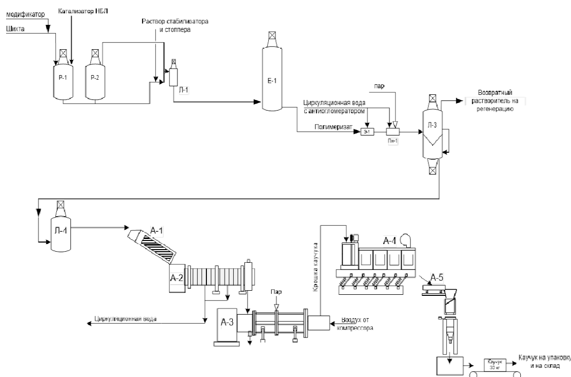
Рисунок 2.1.5 — Принципиальная схема получения СКД-Л
