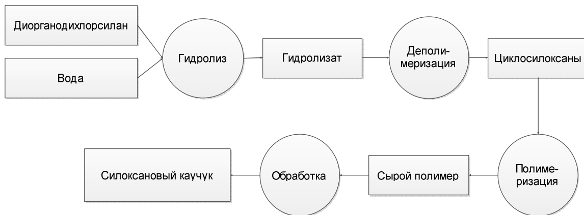
Рисунок 2.3.5 — Принципиальная схема синтеза силоксановых каучуков методом полимеризации
